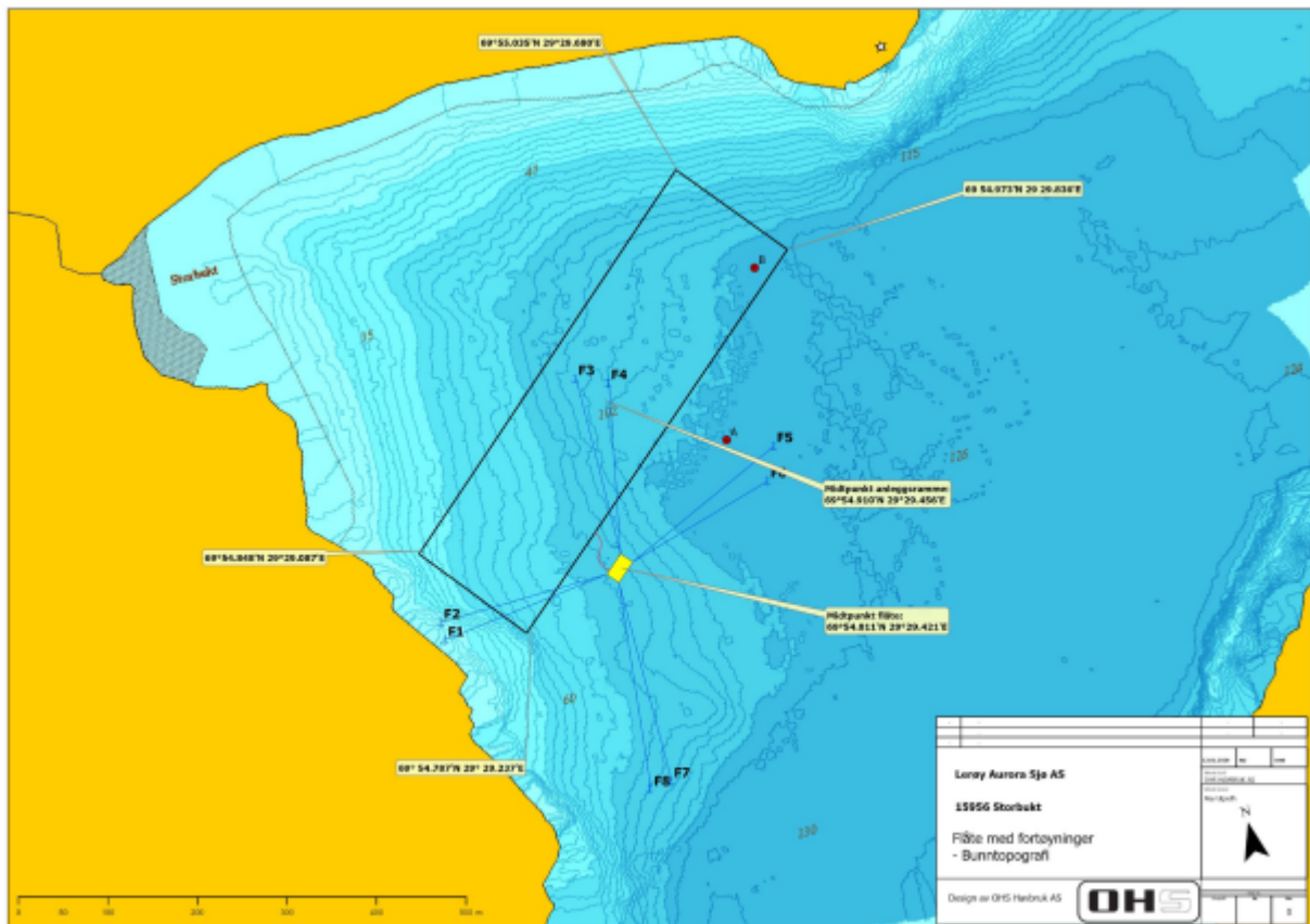
Figur 1 Viser ønsket plassering av flåte (gult rektangel), inkludert åtte fortøyningslinjer med bunnfeste, på lokalitet Storbukt.
